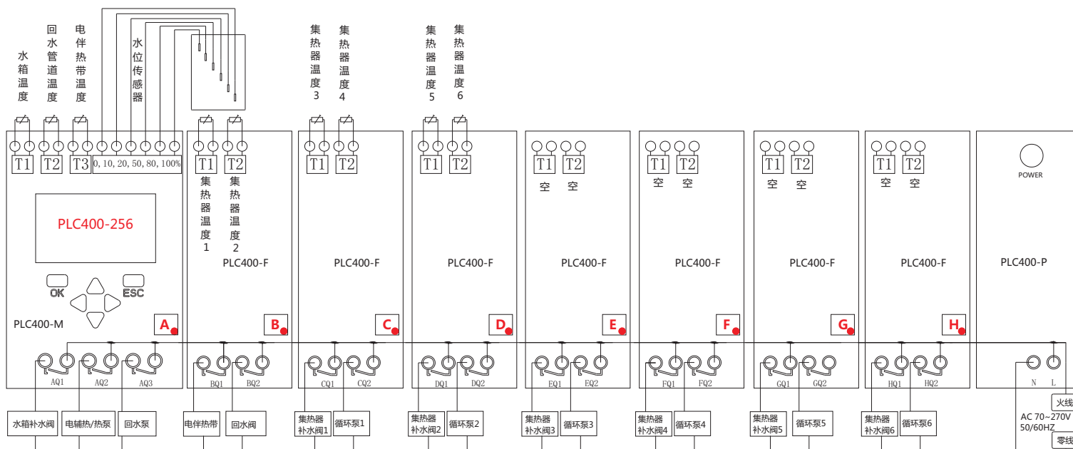
PLC400-256接线示意图
