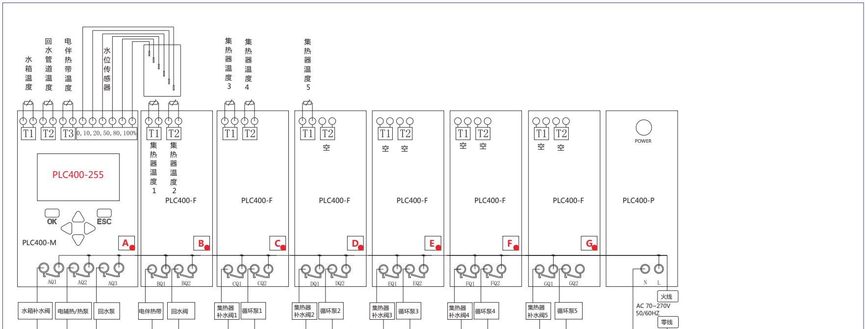
PLC400-255接线示意图
