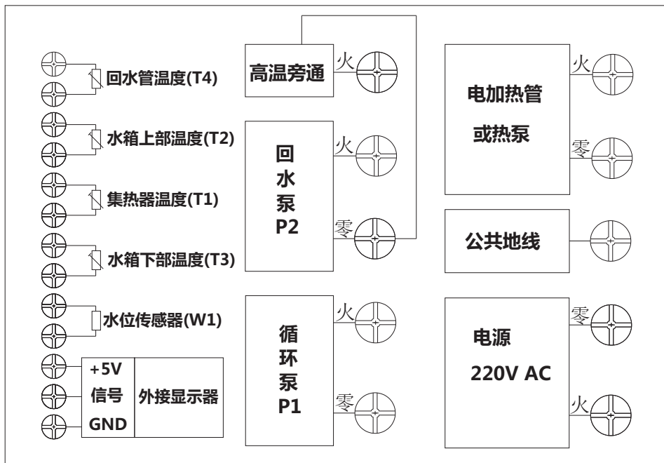
LD-389C2 接线示意图
