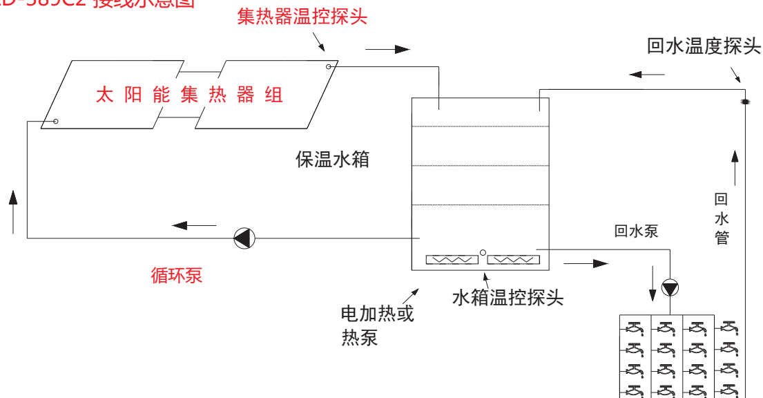
LD-389C2 接线示意图
