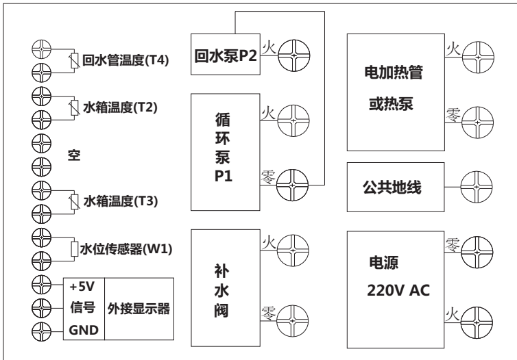
LD-389Q2 接线示意图
