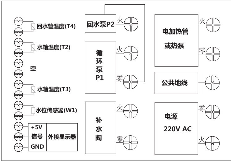
LD-389Q 接线示意图
