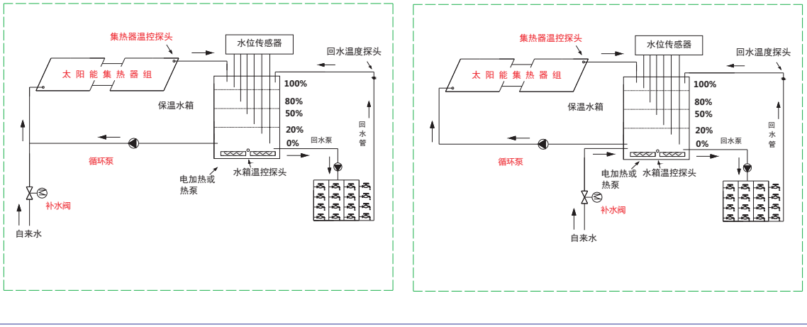
LD-389Q 接线示意图
